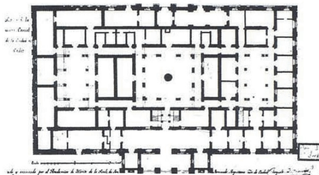
Img. 13.3.- Plano de planta baja de la Cárcel Real
